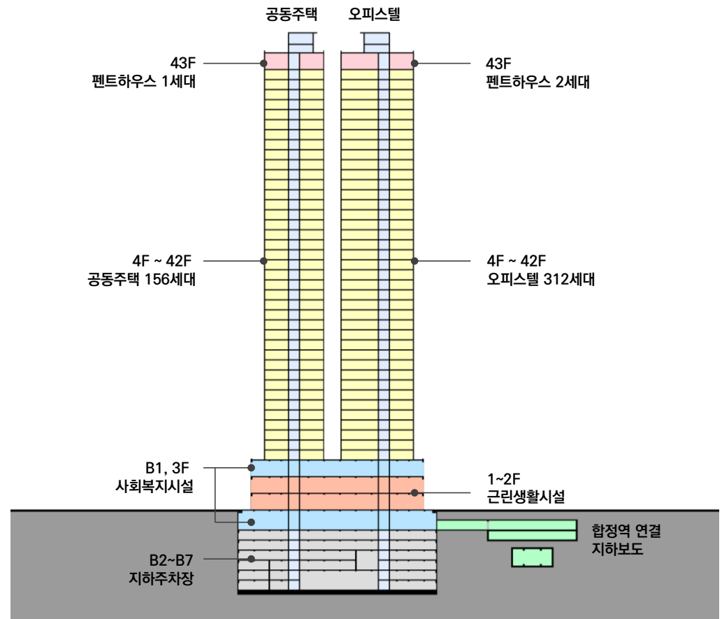
단면도
